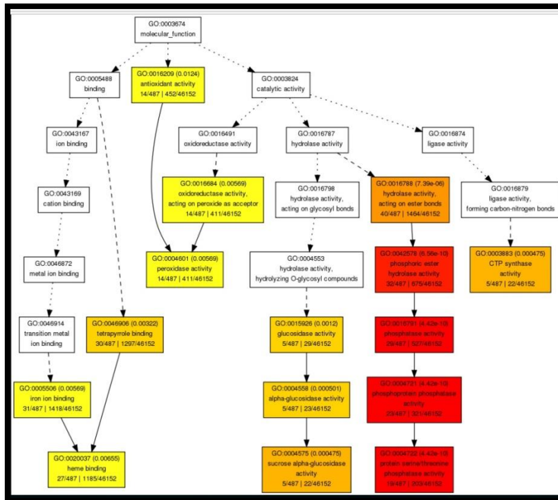
شکل ۲- بخشی از pathway ترسیم شده در رابطه با تجزیه با استفاده از وبسایت AgriGO در سطح معنی داری FDR < 0.05 .
