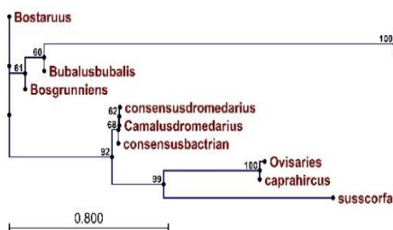
شکل ۲ - ماتریس فواصل ژنتیکی
