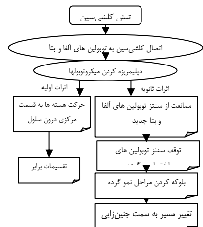
شکل ۶- تنش کلشی سین و مکانیسم های پیشنهاد شده
