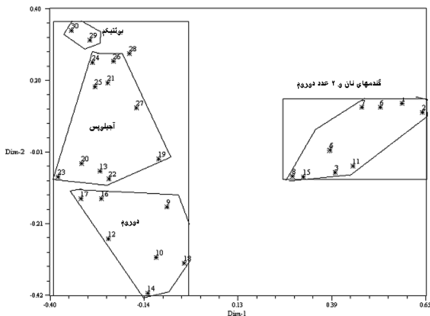
شکل ۴- گروه‌بندی ژنوتیپ‌ها بر اساس ۲ مؤلفه در تجزیه به مؤلفه‌های اصلی (PCoA). چند ضلعی‌ها نشان‌دهنده چهار گروه در تشابه ۰/۷ و مربع مستطیل‌ها نشان‌دهنده دو گروه در تشابه ۰/۶۵ می‌باشد که با گروه‌بندی حاصل از تجزیه کلاستر تقریباً مطابقت می‌کند. شماره‌های نمونه‌ها براساس جدول ۱ می‌باشد.
