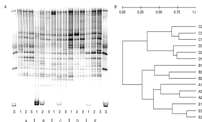
شکل ۴- استفاده از الگوی قطعات تکثیر شده جامعه میکروبی نمونه های گوناگون محیطی در بررسی روابط فیلوژنتیکی میکروبیهای موجود در آنها
