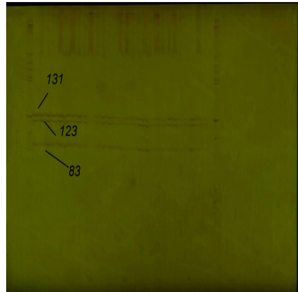
شکل ۳- محصول PCR هضم شده اکزون ۳ ژن میوستاتین توسط آنزیم محدودالایتر HaeIII در چندین نمونه از گوسفندان قره‌گل
