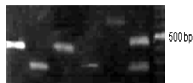
شکل ۴- بیان ژن PtGSP1 در دو مرحله زندگی زنگ برگ گندم به روش RT-PCR. ستون ۱) تکثیر ژن PtGSP1 از روی cDNA حاصل از اسپور جوانه زده؛ ستون ۲) تکثیر ژن توپولین از روی cDNA حاصل از اسپور جوانه زده؛ ستون ۳) تکثیر ژن PtGSP1 از روی cDNA حاصل از مکینه؛ ستون ۴) تکثیر ژن توپولین از روی cDNA حاصل از مکینه؛ ستون ۵) تکثیر ژن PtGSP1 از روی DNA ژنومی حاصل از اسپور جوانه زده؛ ستون ۶) تکثیر ژن توپولین از روی DNA ژنومی حاصل از اسپور جوانه زده. در این تصویر، ستون اول نشان می‌دهد که ژن PtGSP1 در مرحله جوانه‌زنی اسپور قارچ بیان دارد. ستون دوم و چهارم نشان می‌دهد که واکنش سنتز cDNA به درستی انجام شده است به گونه‌ای که cDNA ژن کنترل داخلی توپولین در هر دو مرحله تکثیر شده است. ستون سوم نیز نشان می‌دهد که ژن PtGSP1 در مرحله مکینه نیز بیان دارد. ستون پنجم و ششم نشان می‌دهد آنچه به عنوان cDNA ژن‌ها در ستون‌های اول تا چهارم تکثیر شده ناشی از تکثیر DNA ژنومی ژن PtGSP1 و یا توپولین نبوده است زیرا در این صورت اندازه باندهای تکثیر شده بزرگتر می‌شد.
