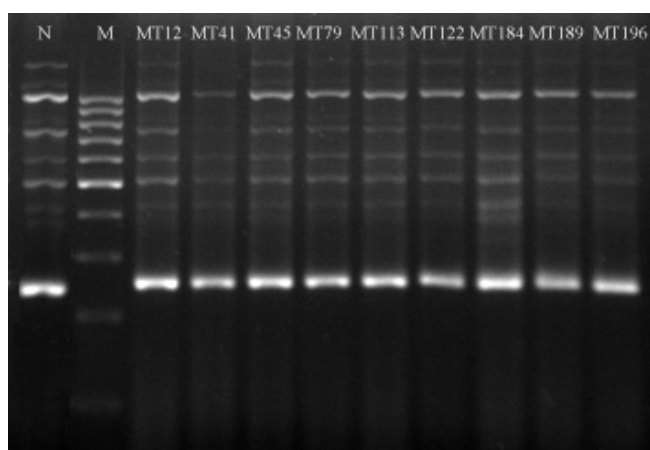
شکل ۳- الگوی باندهای لاین‌های موتانت و رقم شاهد با آغازگر .ISSR6 (N) رقم شاهد (ندا)؛ MT12 تا MT196) لاین‌های موتانت انتخابی؛ (M نشانگر اندازه مولکولی ۱۰۰ bp.
