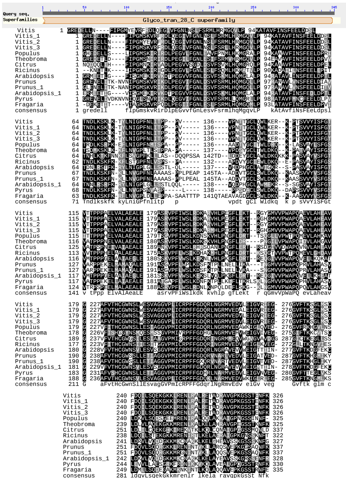
شکل ۲- نمایش دمین حفاظت شده در خانواده UDP - گلوکز: فلاونوئید (UGT) و شباهت سنجی آن در بسیاری از گیاهان نظیر انگور، کاکائو، هلو و آراییدوپسیس و غیره
