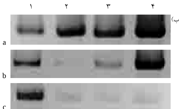
شکل ۴- بررسی بیان ژن PgUGFT در ارقام انار توسط RT-PCR (الف) نمایش کمی بیان ژن PgUGFT در ارقام انار و مراحل رشدی مختلف (۱) گلدی؛ (۲) میوه ابتدای میوه دهی؛ (۳) اواسط میوه دهی؛ (۴) رسیدن میوه، (ب) نمایش محصول PCR روی ژل آگارز یک درصد. (a) پوست سیاه یزد؛ (b) ملس اصفهان؛ (c) شیرین شهاب شیراز و چاهک‌های مراحل رشد (۱) گلدی؛ (۲) میوه ابتدای میوه دهی؛ (۳) اواسط میوه دهی؛ (۴) رسیدن میوه.
