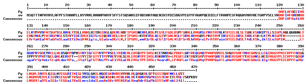
شکل ۵- شباهت سنجی پروتئین PgUFGT و پروتئین UDP-گلوکز: فلاونوئید گلوکز لیز ترانسفراز ، همچنین نمایش شباهت ۵۲ درصدی و حضور اسید آمینه‌های کاملاً یکسان در جایگاه فعال هر دو آنزیم
