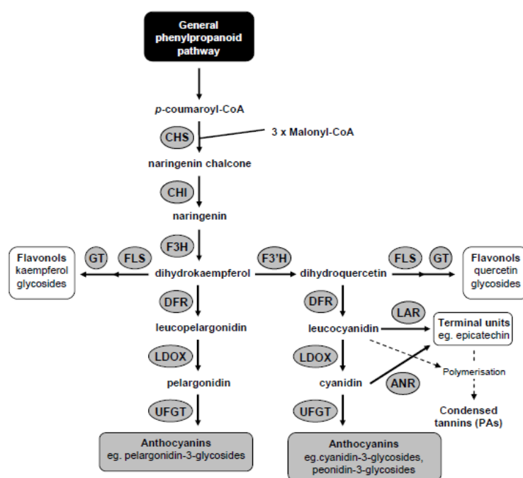
شکل ۱- تصویر کلی مسیر بیوسنتز آنتوسیانین‌ها در گیاهان که منجر به تولید آنتوسیانین می‌شود. CHS) آنزیم چالکون سیتاز؛ F3H) آنزیم فلاونوئید ۳ هیدروکسیلاز؛ DFR) آنزیم دی‌هیدروفلانول ردوکتاز؛ ANS) آنزیم آنتوسیانین سیتاز؛ UFGT) آنزیم UDP-گلوگز: فلاونوئید ۳-O گلوکوزیل ترانسفراز.
