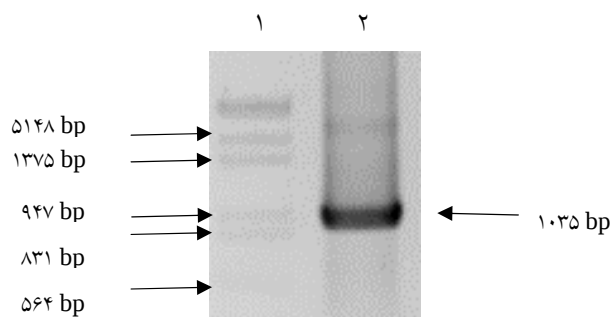
شکل ۳- قطعه تکثیر شده PgUGFT ؛ چاهک (۱) نشانگر اندازه III؛ چاهک (۲) تکثیر قطعه DNA به طول ۱۰۳۵ جفت باز با الگوی cDNA و آغازگرهای UDP-F و UDP-R
