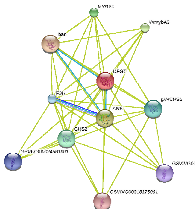
شکل ۷- شبکه ژنی پیش بینی شده ژن VvUFGT در مسیر بیوسنتز آنتوسیانین در انگور (ExPASy (www.ExPASy.org))
