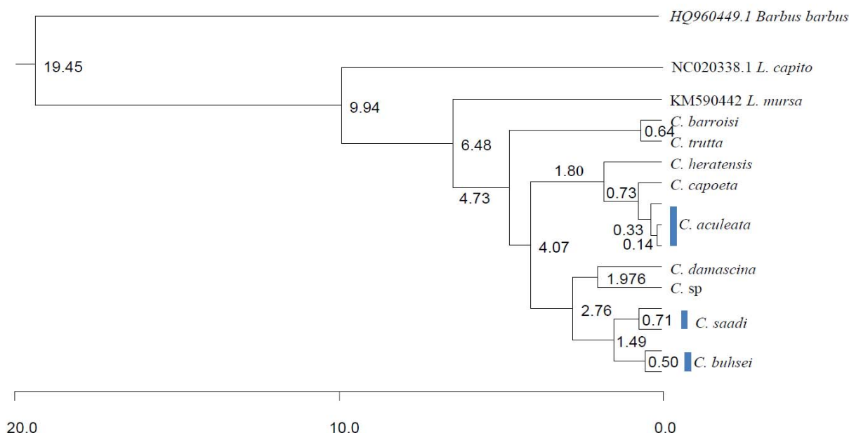
شکل ۴ - ساعت مولکولی ترسیم شده برپایه اطلاعات فسیلی. اعداد در محل گره‌ها نشان‌دهنده زمان محاسبه شده برای جدایی شاخه‌ها بر پایه میلیون سال هستند. خط افقی پایین شکل نشان‌دهنده مقیاس زمانی از زمان صفر (حال حاضر) تا ۲۰ میلیون سال قبل است.
