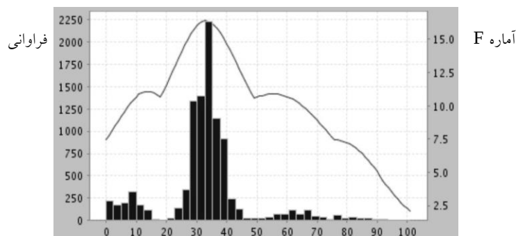
شکل ۱- نمودار ستونی موقعیت QTL را بر روی کروموزوم یک مشخص می‌کند. این نمودار منحنی آماره F را نشان می‌دهد. خط افقی بالا و پایین فراوانی موقعیت QTL را در ده هزار نمونه بوت‌استرپ روی کروموزوم یک برای صفت وزن تولد به ترتیب برای سطوح معنی‌دار پنج و یک درصد را نشان می‌دهند.
