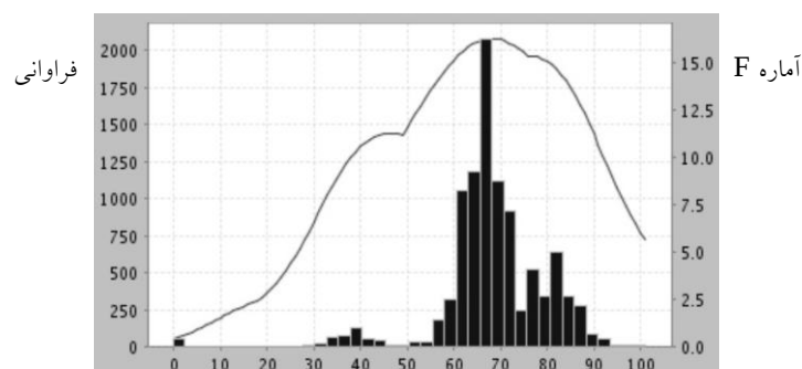
شکل ۳- نمودار ستونی موقعیت QTL را بر روی کروموزوم یک مشخص می‌کند. خط افقی بالا و پایین فراوانی موقعیت QTL را در ده هزار نمونه بوت‌استرپ روی کروموزوم یک برای صفت وزن شش ماهگی به ترتیب برای سطوح معنی‌دار پنج و یک درصد را نشان می‌دهند.
