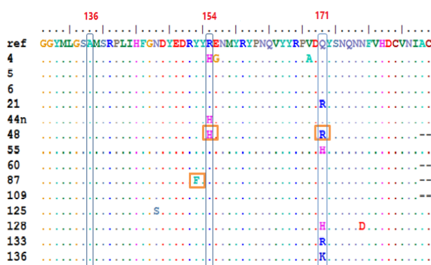
شکل ۴- نتایج تجزیه توالی پروتئینی ژن پرایون گوسفندی در جایگاه اگزون ۳
