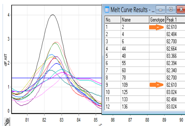
شکل ۳- نمونه‌ای از تعیین ژنوتیپ حاصل از آنالیز منحنی ذوب اگزون سه ژن پرایون گوسفندی، نمونه‌های ۱۰۹ و ۲ دارای پیک یکسان هستند.
