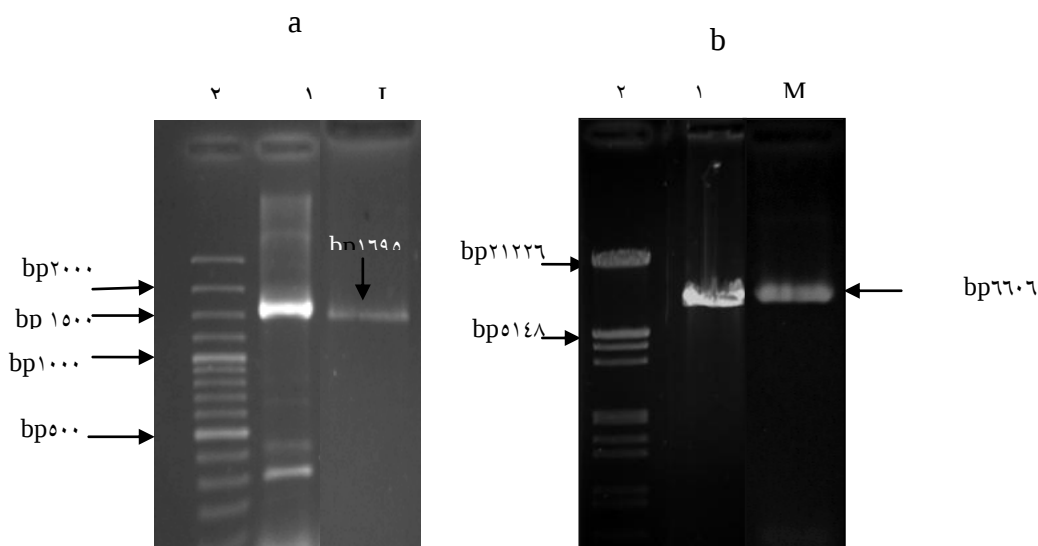
شکل ۴- روند آماده‌سازی ژن LIS و پلاسمید pESC-URA بر روی ژل آگارز. (a) ستون ۱: الکتروفورز محصول PCR ژن LIS ، ستون ۲: خالص‌سازی محصول PCR ژن LIS ؛ (b) ستون ۱: پلاسمید pESC-URA خطی شده با دو آنزیم XhoI و BamHI ، ستون ۲: محصول خالص‌سازی پلاسمید pESC-URA خطی شده از روی ژل، M - نشانگر مولکولی III (فرمنتاس)، (100-3000 bp) DNA Ladder؛ L
