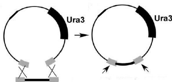
شکل ۵- تکنیک ترمیم شکاف در مخمر ساکارومایسس سرویزیه
