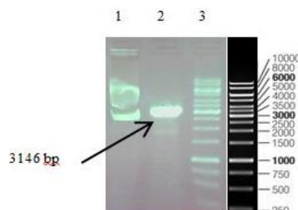
شکل ۶- استخراج DNA پلاسمیدی و برش آنزیمی. ۱- پلاسمید حاوی ژن مورد نظر (قطعه سنس) بدون برش آنزیمی، ۲- محصول برش آنزیمی شامل قطعه ۳۱۴۶ نوکلئوتیدی، ۳- نشانگر وزنی مولکولی (۱ kb DNA - شرکت فرمنتاز).
