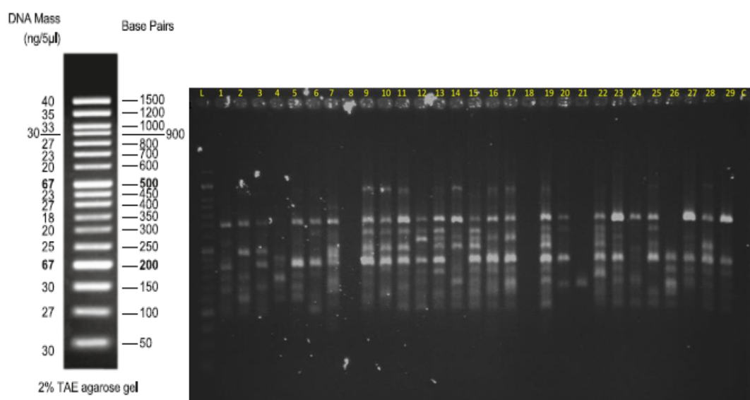
شکل ۱- الگوی نواریابی آغازگر UBC-826 در ژل آگارز ۱/۳ درصد و اندازه مارکر 50bp
