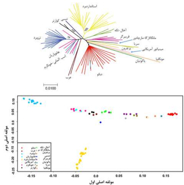
شکل ۱- نمایش ارتباط ژنتیکی میان نژادهای اسب مورد بررسی با استفاده از روش اتصال مجاورین (NJ) و تحلیل مؤلفه‌های اصلی با استفاده از داده‌های توالی‌یابی مربوط به نژادهای مختلف اسب
