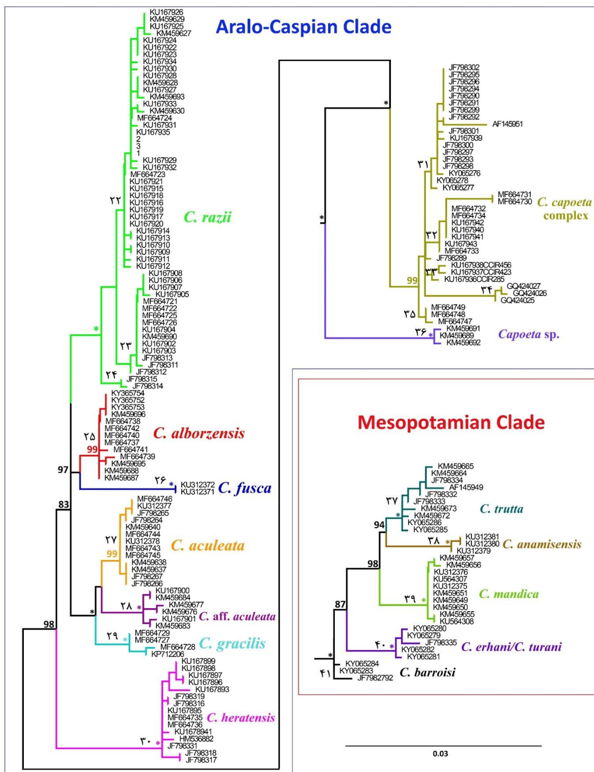
شکل ۳- درخت تبارشناسی شاخه‌های آرال-کاسپین و بین‌النهرین اعضای مورد بررسی جنس Capoeta با استفاده از نرم‌افزار IQ-TREE (اعداد روی گره‌ها میزان UFBoot2 است. در صورت کامل بودن UFBoot2 در گره از ستاره * استفاده شد).
