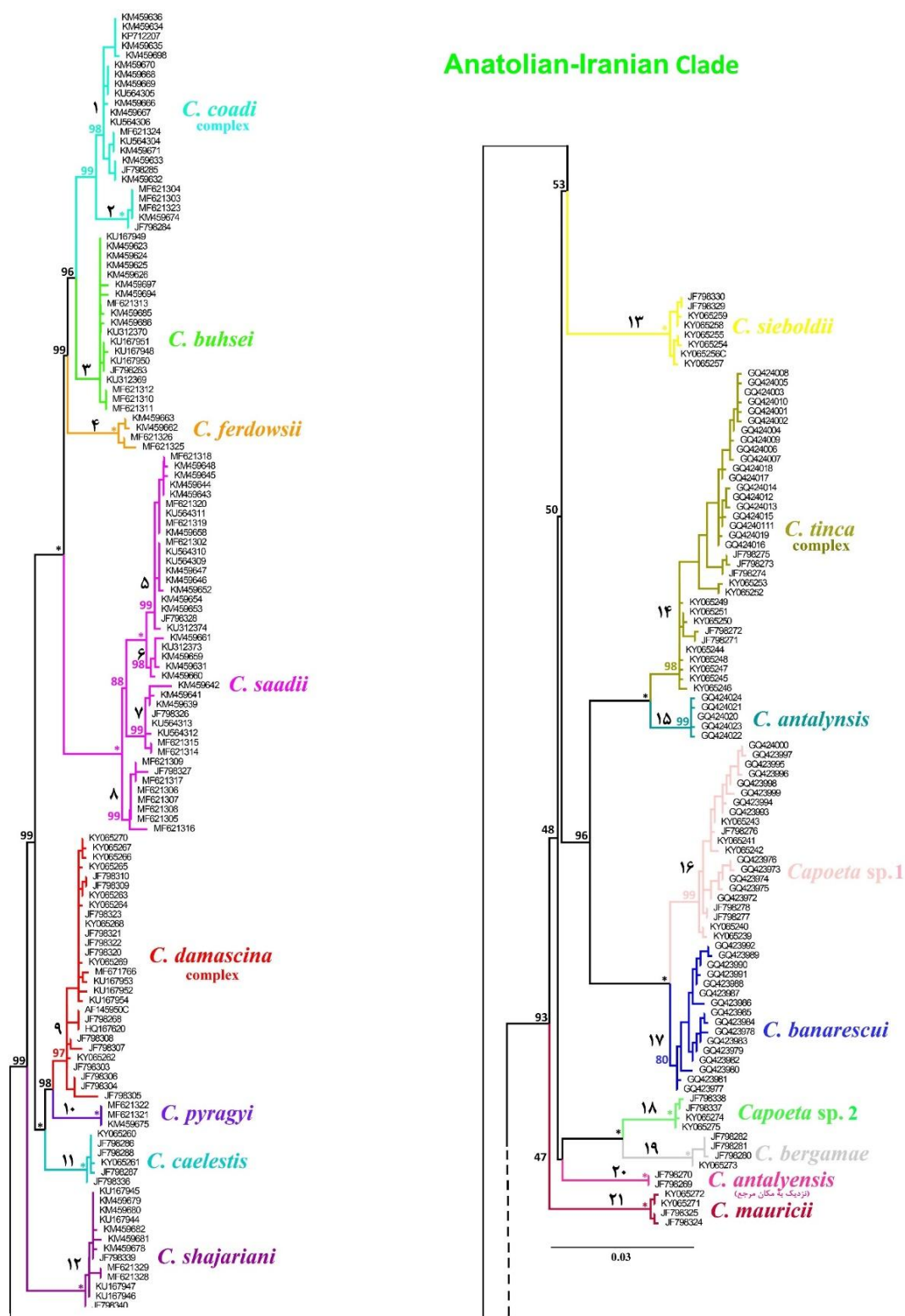
شکل ۲- درخت تبارشناسی شاخه ایران-آناتولی اعضای مورد بررسی جنس Capoeta با استفاده از نرم افزار IQ-TREE (اعداد روی بازوها میزان UFBboot2 است، در صورت کامل بودن UFBboot2 در گره از ستاره * استفاده شد).
