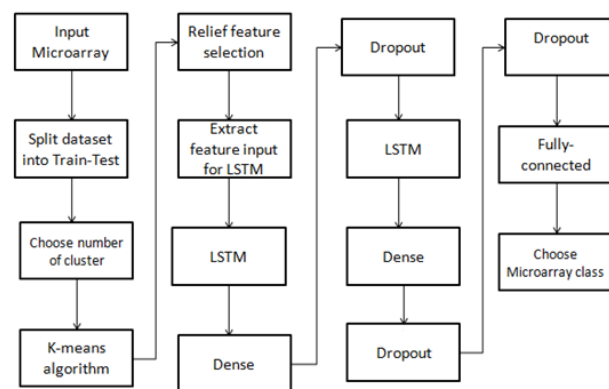
شکل ۴- فلوچارت روش پیشنهادی
