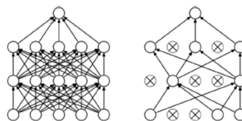
شکل ۳- نحوه عملکرد لایه حذف تصادفی (Gal and Ghahramani 2016)
