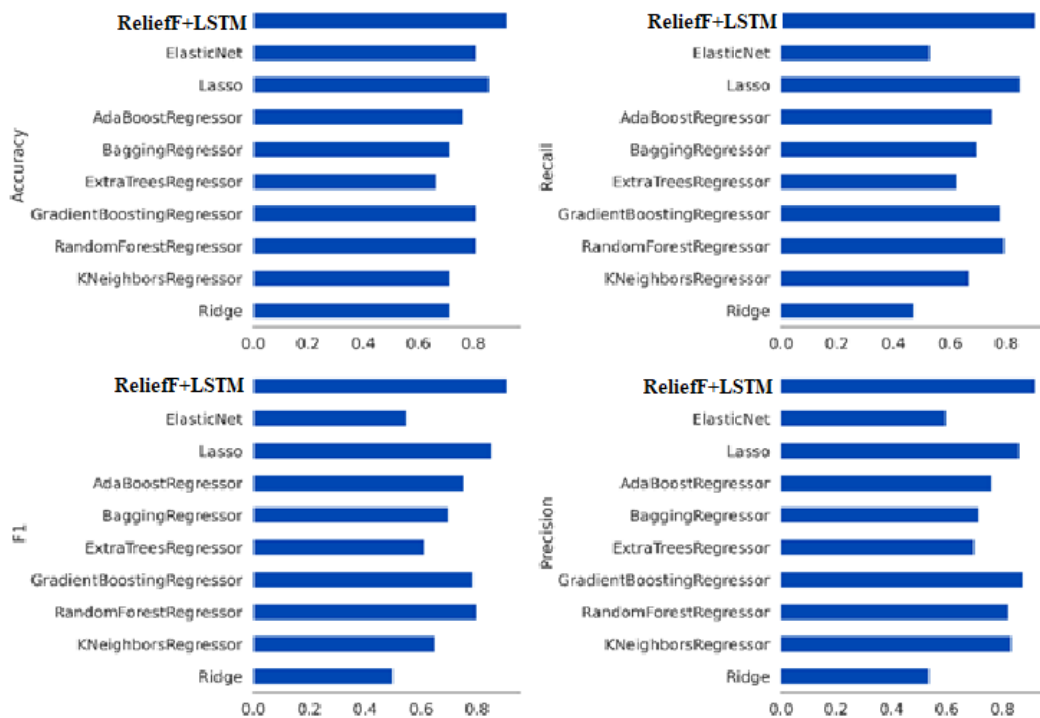
شکل ۷- مقایسه روش پیشنهادی با ۹ الگوریتم دیگر در مجموعه داده کلوئکتال
