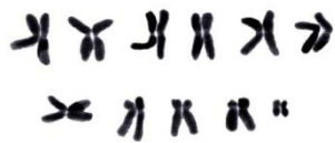
فریدونشهر (2n=22)
