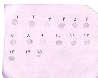
شکل ۱۰- آزمون لکه‌گذاری گندم تراریخته برای پیشبر CaMV35S نمونه‌های ۱-۱۳. گیاهچه‌های تراریخته لاین A، نمونه ۱۴. گیاه شاهد (کنترل منفی)، نمونه ۱۵. پلاسمید (کنترل مثبت) آزمون لکه‌گذاری DNA، حضور ژن نومایسین فسفوترانسفراز و پیشبر CaMV35S را در ۱۵ گیاهچه تراریخته تایید کرد.
