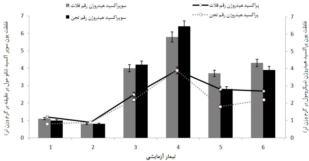
شکل ۴- تغییرات میزان رادیکال‌های سوپر اکسید و پراکسید هیدروژن ۴۸ ساعت پس از اعمال تیمارهای آزمایشی شامل محلول پاشی: ۱) آب (شاهد) ۲) اسید اسکوربیک (۲۰ میلی مولار) ۳) نیترات نقره (۰/۷۵ میلی مولار) ۴) نیترات نقره (۱/۵ میلی مولار) ۵) تیمار ترکیبی اسید اسکوربیک (۲۰ میلی مولار) + نیترات نقره (۰/۷۵ میلی مولار) ۶) تیمار ترکیبی اسکوربیک (۲۰ میلی مولار) + نیترات نقره (۱/۵ میلی مولار). مقدار خطای معیار (n=۴) برای هر میانگین به طور جداگانه نشان داده شده است.
