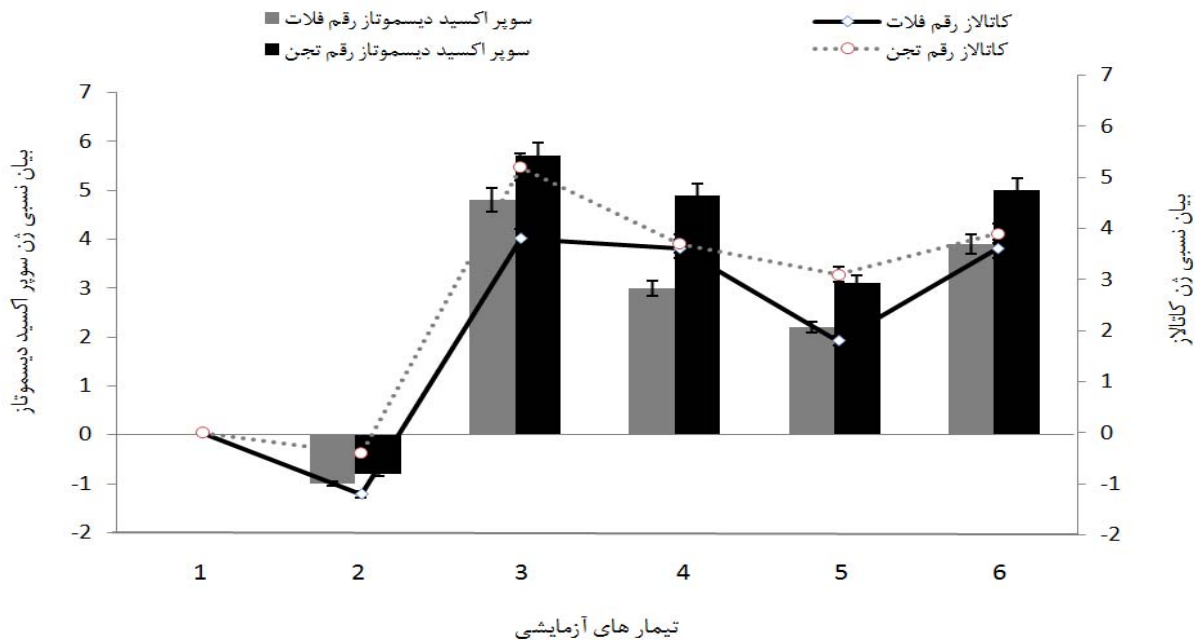
شکل ۵- تغییرات بیان ژن‌های سوپراکسید دیسموتاز و کاتالاز ۱۰ ساعت پس از اعمال تیمارهای آزمایشی شامل محلول پاشی: (۱) آب (شاهد) (۲) اسید اسکوربیک ۲۰ میلی مولار (۳) نیترات نقره ۰/۷۵ میلی مولار (۴) نیترات نقره ۱/۵ میلی مولار (۵) تیمار ترکیبی اسید اسکوربیک (۲۰ میلی مولار) + نیترات نقره (۰/۷۵ میلی مولار) (۶) تیمار ترکیبی اسکوربیک (۲۰ میلی مولار) + نیترات نقره (۱/۵ میلی مولار). مقدار خطای معیار ( n=4 ) برای هر میانگین به طور جداگانه نشان داده شده است.
