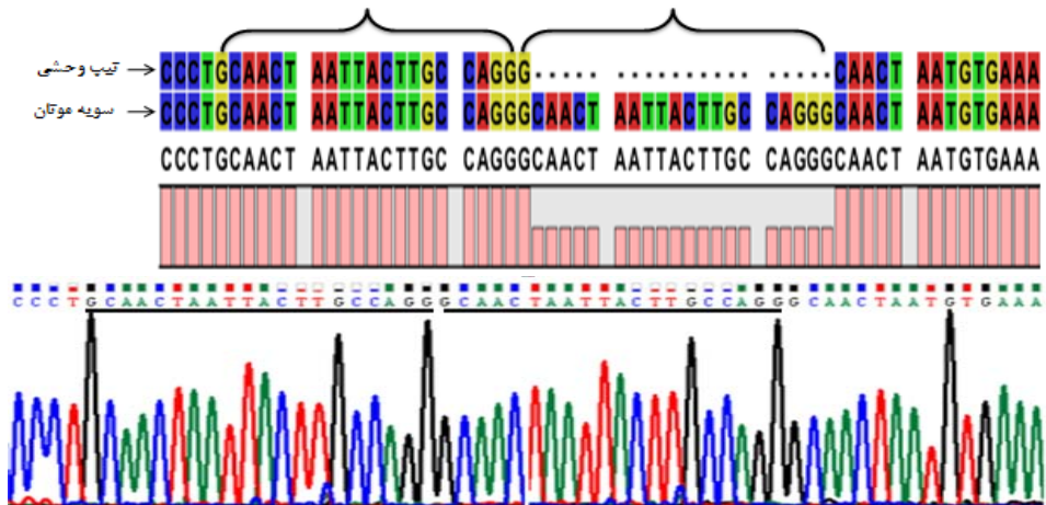
شکل ۳- تکرار ۲۰ جفت باز (GCAACTAATTACTTGCCAGG) در اپراتور marO نتیجه حاصل از بررسی همولوژی بین تیپ وحشی و سویه موتان با استفاده از نرم‌افزار CLC (تغییر حاصله به صورت کروشه) و منحنی کروماتوگرام مربوطه (تغییر حاصله به صورت خط در زیر ناحیه تغییر یافته).
