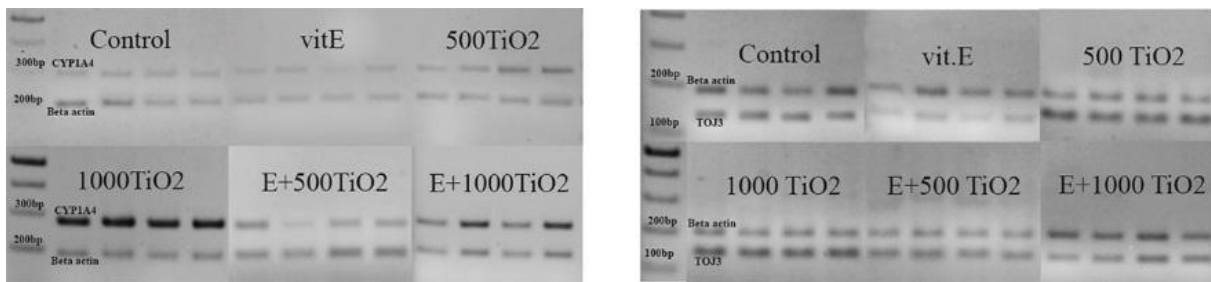
شکل ۱- بیان ژن CYPIA4 در سمت چپ و ژن TOJ3 در سمت راست در تیمارهای مختلف نسبت به ژن مرجع بتا اکتین نشان داده شده است.
