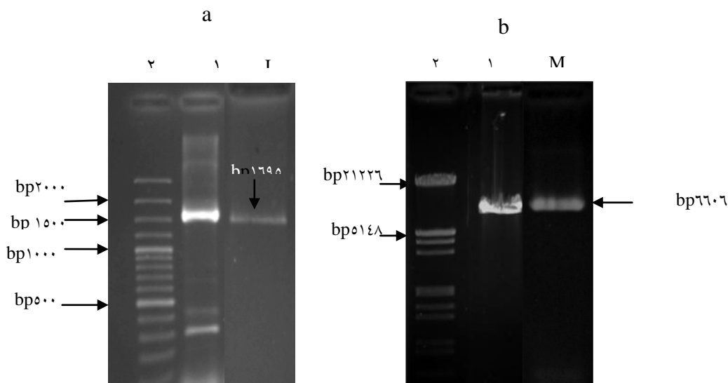
شکل ۴- روند آماده‌سازی ژن LIS و پلاسمید pESC-URA بر روی ژل آگارز. (a) ستون ۱: الکتروفورز محصول PCR ژن LIS، ستون ۲: خالص‌سازی محصول PCR ژن LIS؛ (b) ستون ۱: پلاسمید pESC-URA خطی شده با دو آنزیم XhoI و BamHI ، ستون ۲: محصول خالص‌سازی پلاسمید pESC-URA خطی شده از روی ژل، M - نشانگر مولکولی III (فرمنتاس)، (۱۰۰-۳۰۰۰ bp) DNA Ladder: L.
