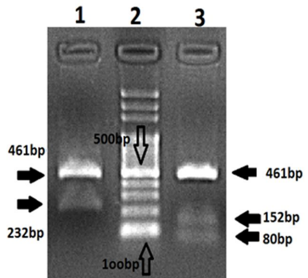
شکل ۲- الکتروفورز محصولات PCR پلی مورفیسم اینترون ۱۹ پس از هضم با آنزیم HindIII بر روی ژل آگاروز سه درصد؛ چاهک ۱، مرد همی زیگوت C (negative)؛ چاهک ۳، مرد همی زیگوت T (positive)؛ چاهک ۲، 100 bp ladder
