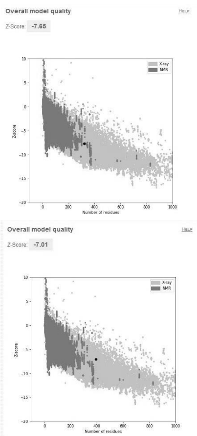
شکل ۵- نقشه Z-score و سایت Prosa. Z-score کیفیت کلی مدل را نشان می‌دهد و به‌وسیله کریستالوگرافی اشعه X (روشن) یا اسپکتروسکوپی NMR (تیره) با توجه به طول زنجیره‌های پروتئینی موجود در پایگاه PDB تعیین می‌شود. Z-score پروتئین Q65F56 به‌صورت یک نقطه بزرگ مشخص شده است.
