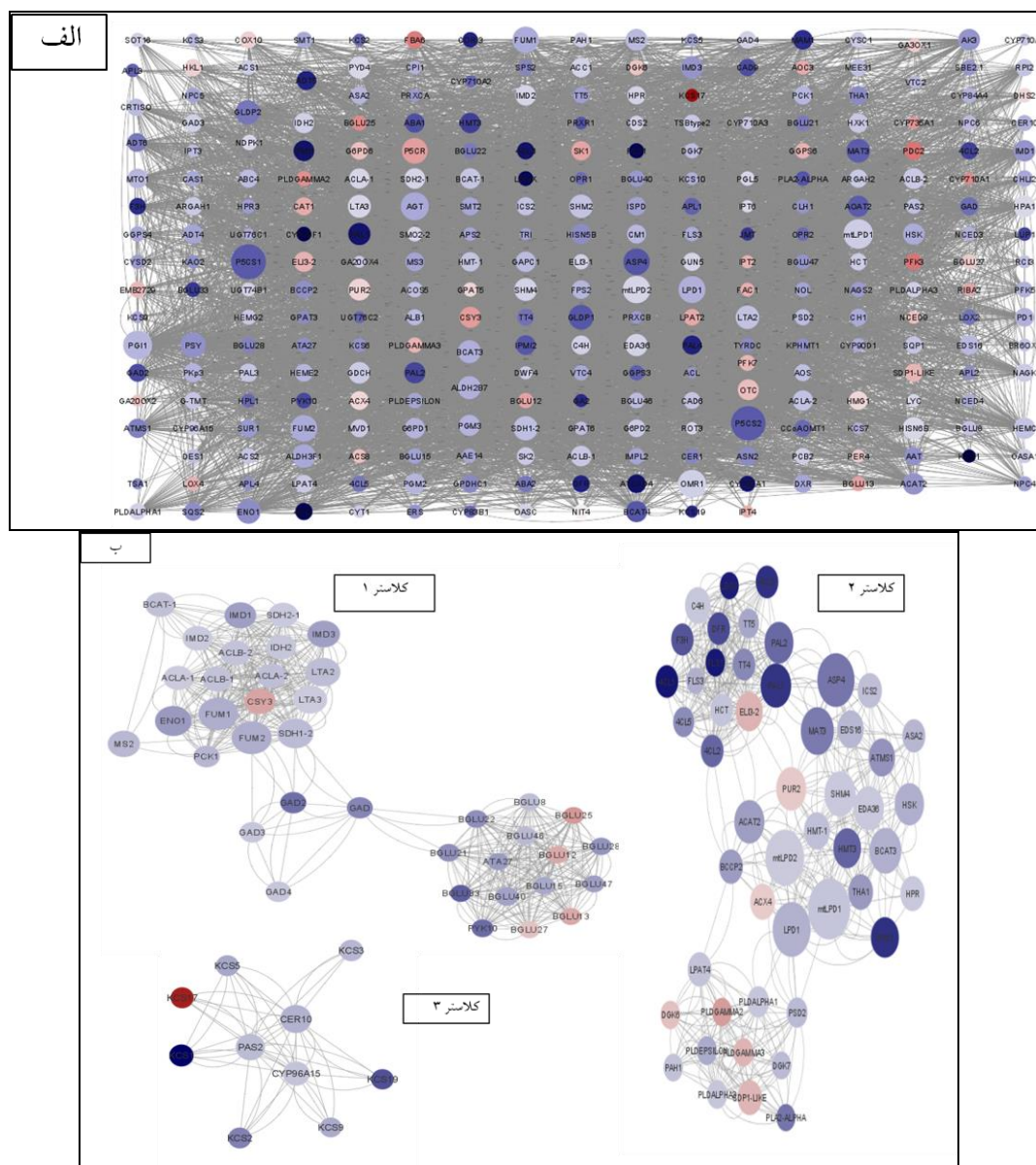
شکل ۵-الف. شبکه‌ی مرتبط با ژن‌های در ارتباط با مسیر بیوسنتز متابولیت‌های ثانویه و ب. کلاسترهای این شبکه
