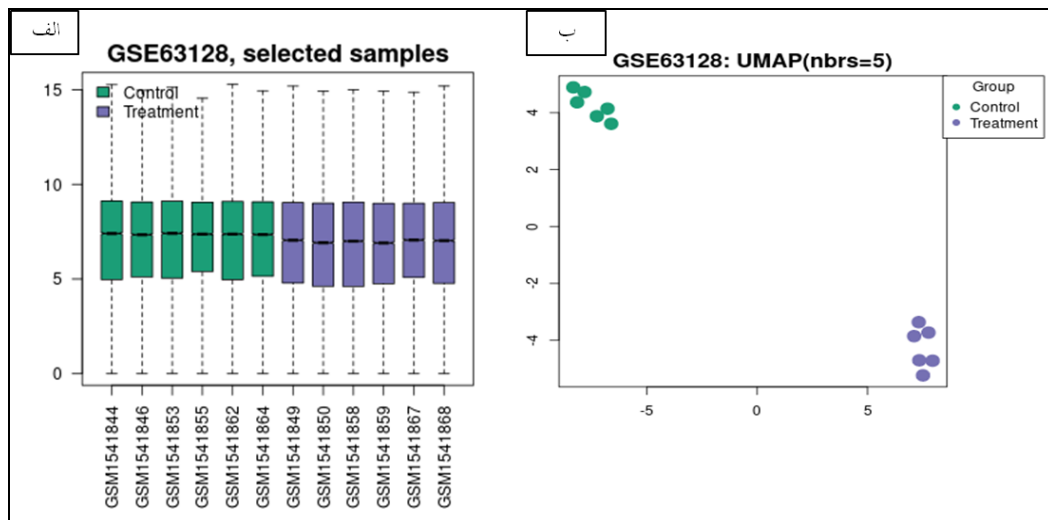
شکل ۱- الف. نمای شماتیک از نمودار جعبه‌ای نحوه‌ی توزیع مقادیر نمونه‌های مورد استفاده پس از نرمال‌سازی ب. نمای شماتیک از نمودار بررسی تنوع بر اساس آنالیز PCA
