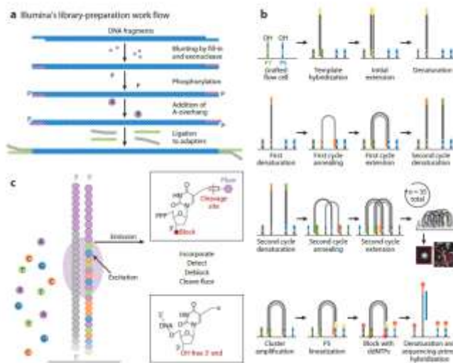
شکل ۲- مقایسه روش‌های توالی‌یابی سنگر و ایلومینا. توالی‌یابی سنگر (A)، توالی‌یابی ایلومینا (B). فرآیند ساخت کتابخانه ایلومینا (a)، تولید کلاستر ایلومینا از طریق تکثیر پل (b)، توالی‌یابی ایلومینا از طریق سنتز با پایانه‌های رنگ برگشت پذیر (c)
