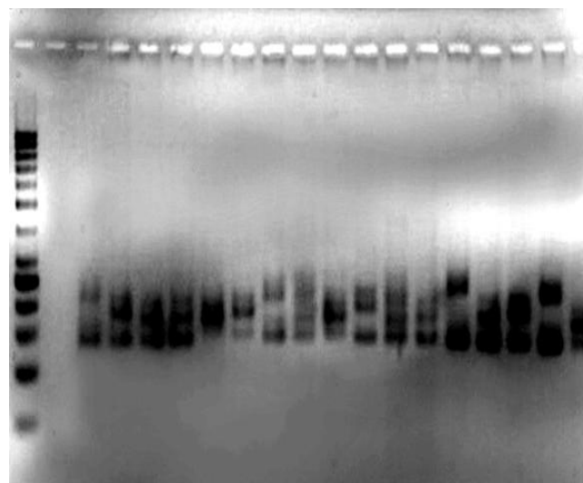
شکل ۱- مکان ریزماهوره تکثیر شده (لوکوس xgwm33-1d)
