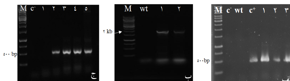
شکل ۳- الف) نتایج PCR بر روی گیاهان باززا شده برای تأیید انتقال ژن اینترفرون گاما به ژنوم کلروپلاست توتون با استفاده از آغازگرهای F1 و R. M نشانگر 1 kb؛ C - کنترل منفی؛ wt گیاه شاهد؛ C + کنترل مثبت؛ (۱-۳) گیاهان تراریخت کلروپلاستی ب) نتایج PCR برای تأیید درج ژن اینترفرون گاما در محل صحیح درون ژنوم کلروپلاست با استفاده از آغازگرهای F3 و R. M نشانگر 1 kb؛ wt گیاه شاهد؛ (۱-۲) گیاهان تراریخت کلروپلاستی ج) نتایج RT-PCR. M نشانگر 1 kb؛ C - کنترل منفی؛ (۱) RNA کل بعد از تیمار با DNase؛ (۲) کنترل مثبت؛ (۳-۵) cDNA به عنوان الگوی PCR.
