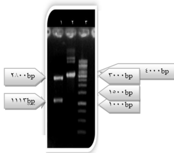
شکل ۱- الکتروفورز محصول برش آنزیمی پلاسمید نو ترکیب pKGH-Ta3 با آنزیم های Xba I و Pst I ؛ چاهک ۱) محصول برش آنزیمی پلاسمید نو ترکیب؛ چاهک ۲) پلاسمید نو ترکیب بریده نشده؛ چاهک ۳) نشانگر وزن مولکولی DNA (1 kb DNA ladder Fermentas).
