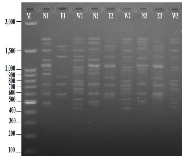
شکل ۲- الگوی باندهای حاصل از تکثیر DNA ژنومی نمونه‌های بومادران توسط آغازگر e3. M نشانگر وزن ملکولی ۱۰۰ bp plus؛ N1، N2 و N3 سه تکرار از نمونه‌های مربوط به شمال استان هرمزگان (حاجی آباد)؛ E1، E2 و E3 سه تکرار از نمونه‌های مربوط به شرق استان هرمزگان (بشاگرد)؛ W1، W2 و W3 نمونه‌های مربوط به غرب استان هرمزگان (پارسیان)
