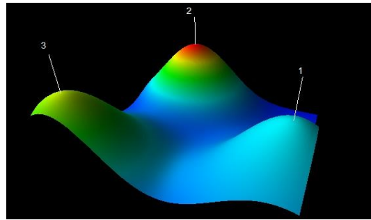
شکل ۴- نمایش قله‌ای حاصل از تجزیه خوشه‌ای به وسیله الگوریتم گروه‌بندی RB با استفاده از نرم‌افزار gCLUTO V1/0؛ ۱. توده حاجی‌آباد (سربرزه)؛ ۲. توده پارسیان (بنجراشک)؛ ۳. توده بشاگرد (سرزرد)
