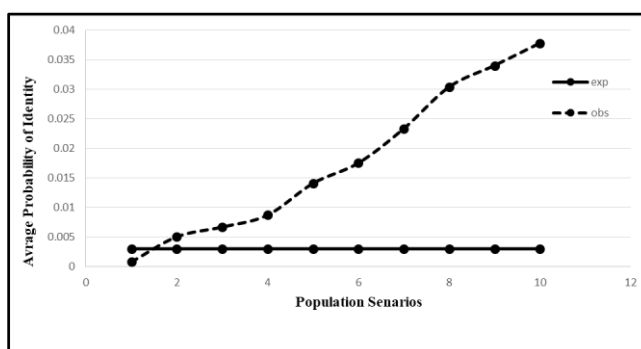
شکل ۴- شاخص احتمال تشابه افراد ( PID ). با افزایش روابط خویشاوندی بین افراد یک جمعیت میزان شاخص PID_{exp} (مورد انتظار) افزایش می‌یابد. شاخص PID_{obs} (مشاهده شده) برای کل سناریوهای در نظر گرفته شده برابر با ۰/۰۰۳ است.
