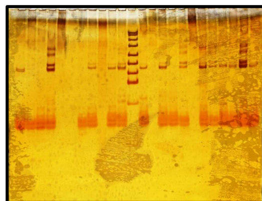
شکل ۲- تصویر ژل آکرل آمید مربوط به یکی از لوکوس‌های تکثیر شده به منظور بررسی تنوع ژنتیکی و روابط خویشاوندی خرس قهوه‌ای
