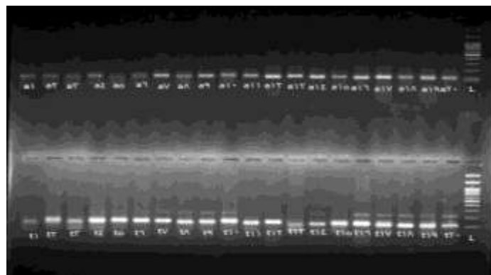
شکل ۱- الگوی باندهای نشانگر SSR (Xgwm-157) در گونه‌های Agilops و Triticum واجد ژنوم D در سطوح مختلف پلوئیدی. L و a و t نشان‌دهنده leader، Ae. tauschii (t) و T. aestivum (a) می‌باشد.
