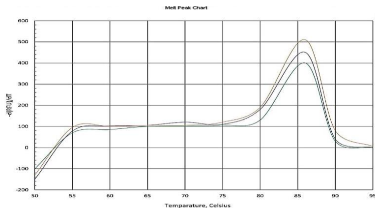
شکل ۲- منحنی ذوب
