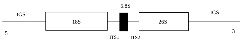
شکل ۲- نمایش شماتیک ساختار rDNA در ژنوم گیاهان
