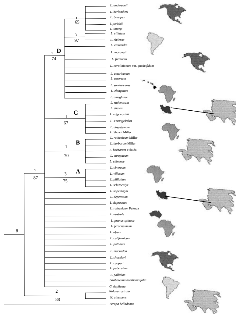
شکل ۶- درخت حداکثر پارسیمونی (با طول ۱۳ گام، RI=10 CI=1 ) برای توالی trnL-trnF در جنس Lycium و Grobowskia و Nolana spp. و Atropa belladonna به عنوان برون گروه استفاده شدند. عدد بالای هر شاخه طول شاخه و عدد پایین آن مقدار بوتسترپ با ۱۰۰ تکرار را نشان می‌دهد. مقادیر <50\% نشان داده نشده است. مناطق جغرافیایی نیز در سمت راست نشان داده شده است.
