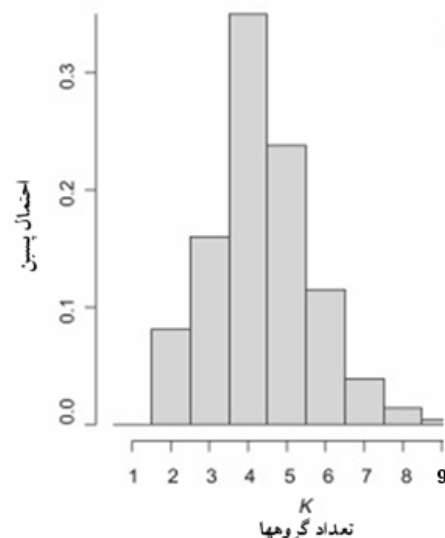
شکل ۳- تعداد گروه‌های همگن (K). تعداد چهار گروه در اینجا حداکثر احتمال را داشته و حداکثر تعداد گروه همگن در نمونه‌های مورد بررسی می‌باشد.
